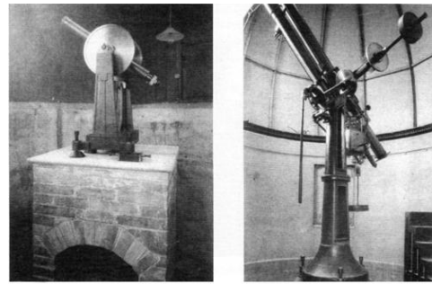
ANTEOJO MERIDIANO Y ANTEOJO ECUATORIAL (OBSERVATORIO)
